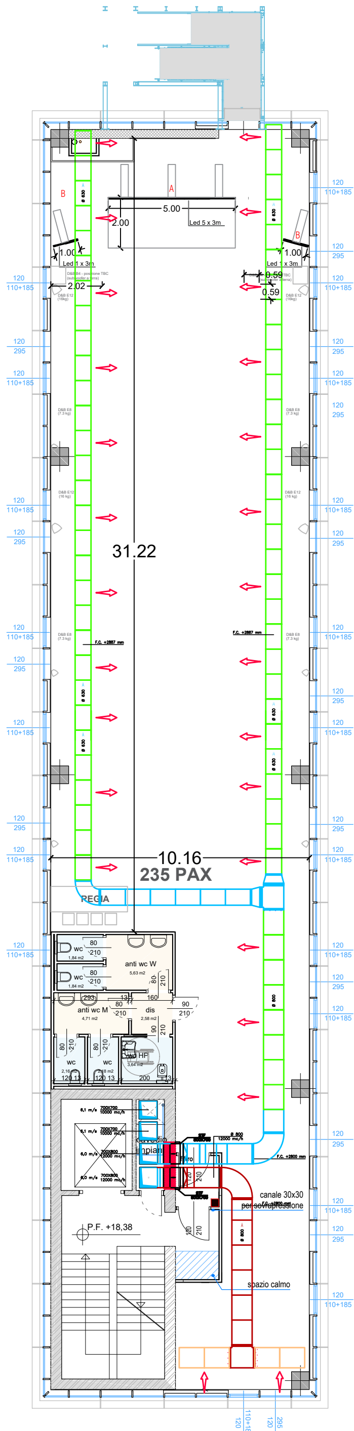
PIANO TERZO
